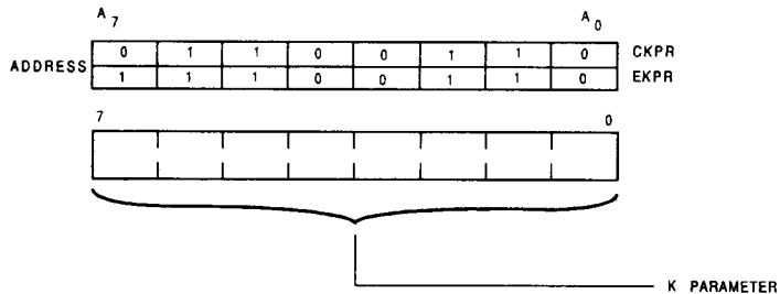
Figure 28. K Parameter Registers (CKPR, EKPR)
